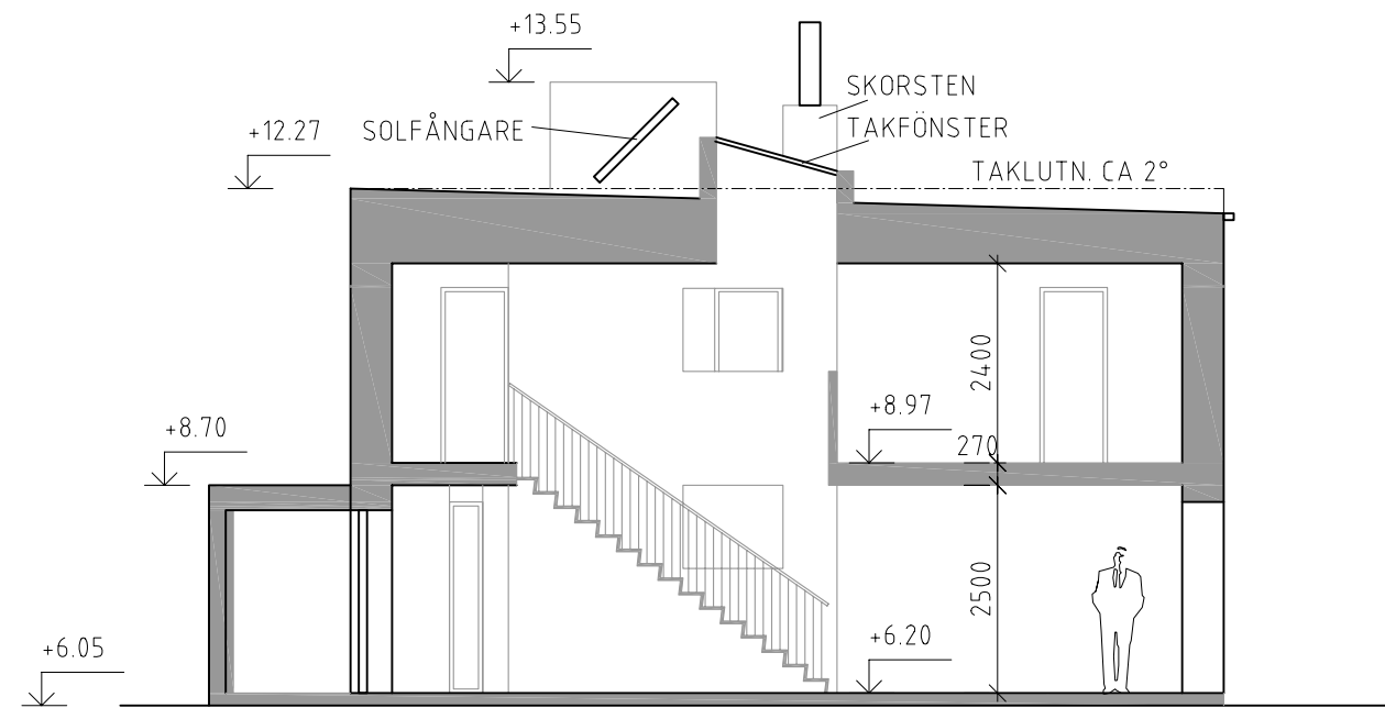
SEKTION A-A (SÖDRA HUSET).
